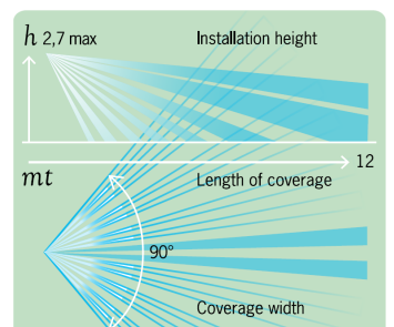
SSL - Optionele Lens voor installatie tussen 2.2 & 2.7m (Alle versies Spectrum behalve WALL)
