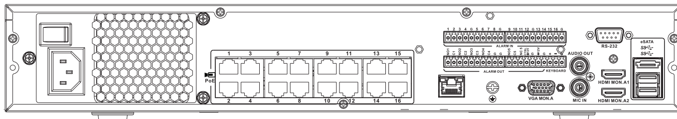
Panneau arrière DIVAR 5000 network (16 PoE)
