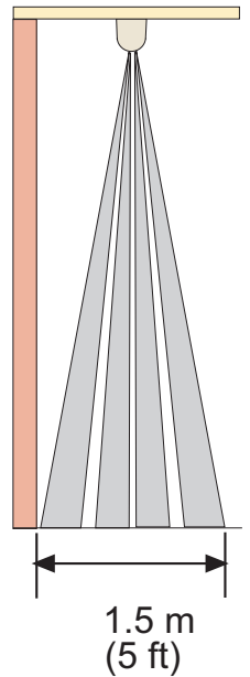
Vue latérale Plus vous montez le détecteur haut, plus la zone de couverture sera large. N'installez pas le DS160/DS161 à plus de 4,6 m du sol. Vue de côté du diagramme de couverture lorsque l'unité est installée à 4,6 m du sol, lentille dirigée vers le bas.
