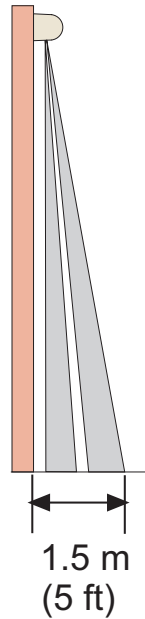
Vue latérale Plus vous montez le détecteur haut, plus la zone de couverture sera large. N'installez pas le DS160/DS161 à plus de 4,6 m du sol.
