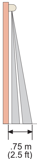
Vue latérale Plus vous montez le détecteur haut, plus la zone de couverture sera large. N'installez pas le DS160/DS161 à plus de 4,6 m du sol. Vue de côté du diagramme de couverture lorsque l'unité est installée à 4,6 m du sol, lentille dirigée vers le bas.
