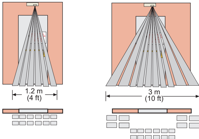
Vue avant Montage mural au-dessus de la porte et montage au plafond à 75 cm devant la porte.
